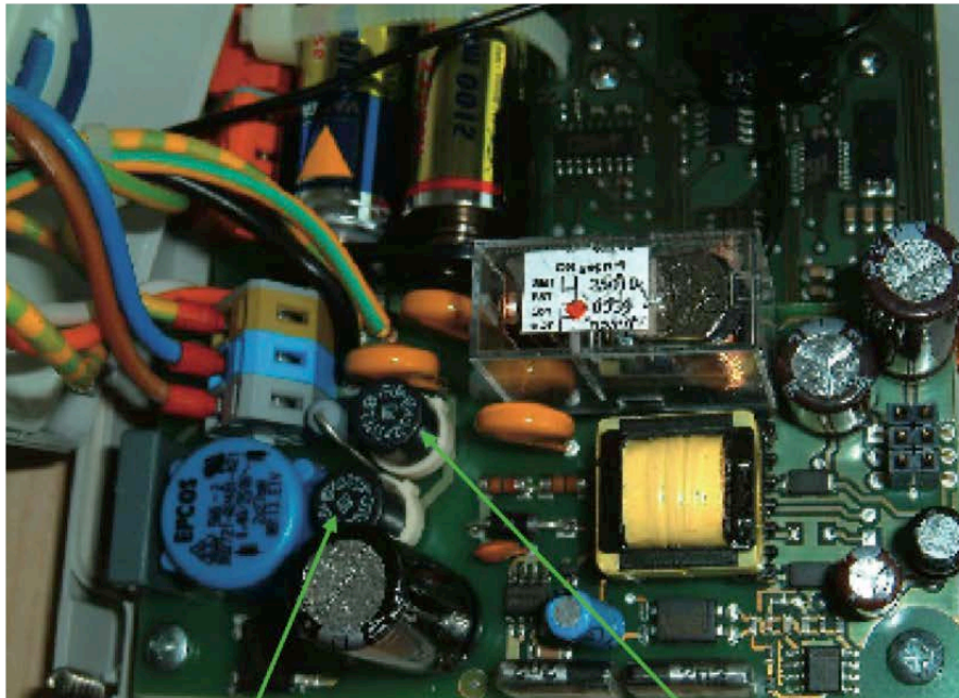
Fusible panneau de commande TR5 ; T0,5A
